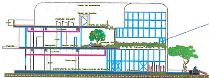
SECCIÓN TRANSVERSAL C-D
